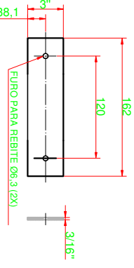
DETALHE ITEM 8
